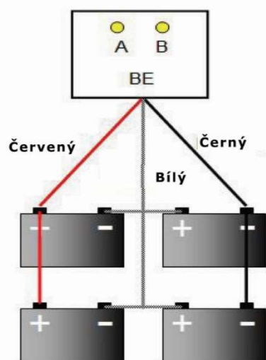
24V sestava ze 4 baterií
