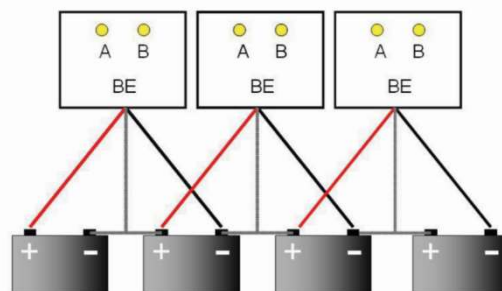
48V bateriová sestava
