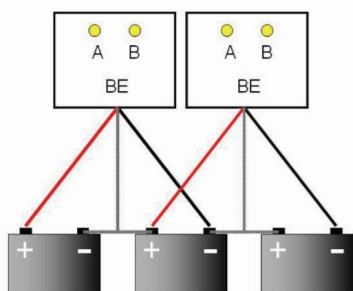
36V bateriová sestava
